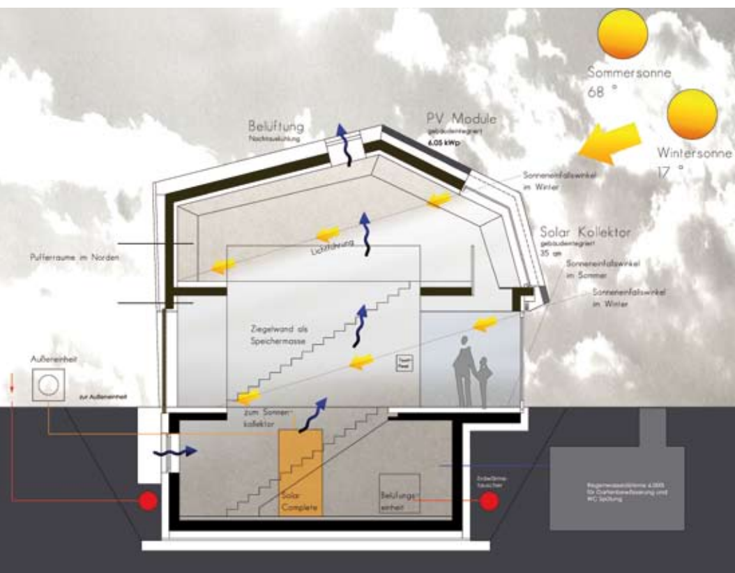
Systemschnitt Solar Aktiv Haus
